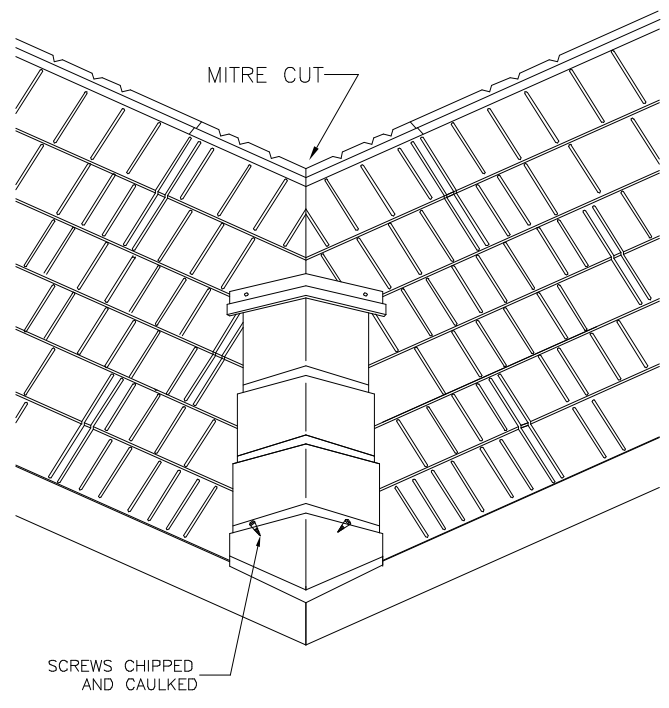
HIP CAP
